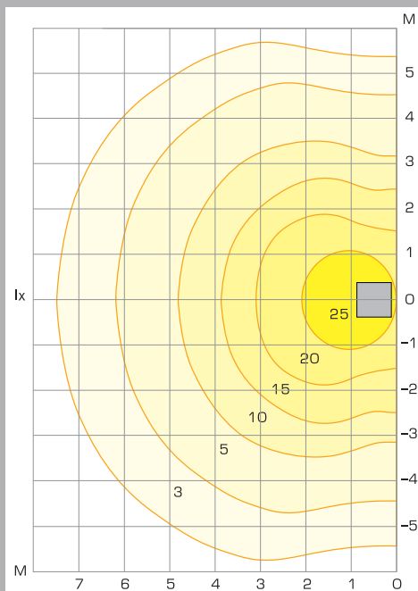
Диаграмма освещенности для SIG 150 Монтажная высота 4 м
