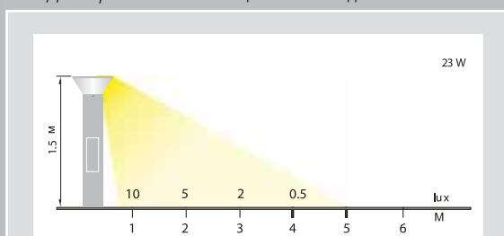
Диаграмма освещенности для SP-23H
