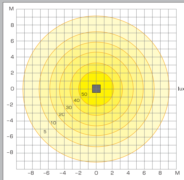
Диаграмма освещенности для IM43/150W Площадь 20 x 20 метров
