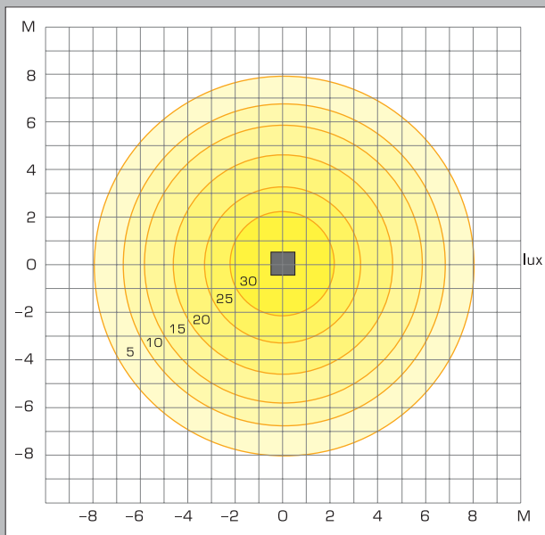
Диаграмма освещенности для IM43/70W Площадь 20 x 20 метров
