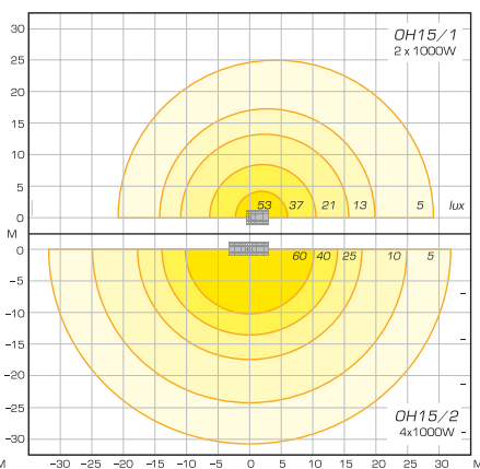
Диаграмма освещенности Площадка 65 x 70 метров
