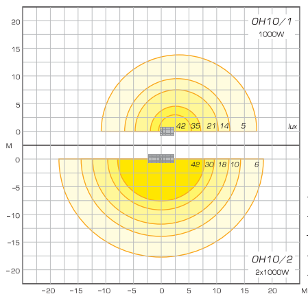
Диаграмма освещенности Площадка 45 x 50 метров
