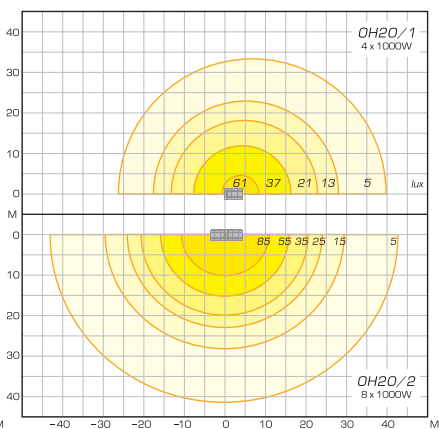
Диаграмма освещенности Площадка 90 x 100 метров
