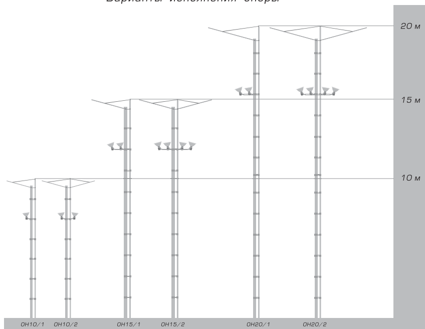
Варианты исполнения опоры
